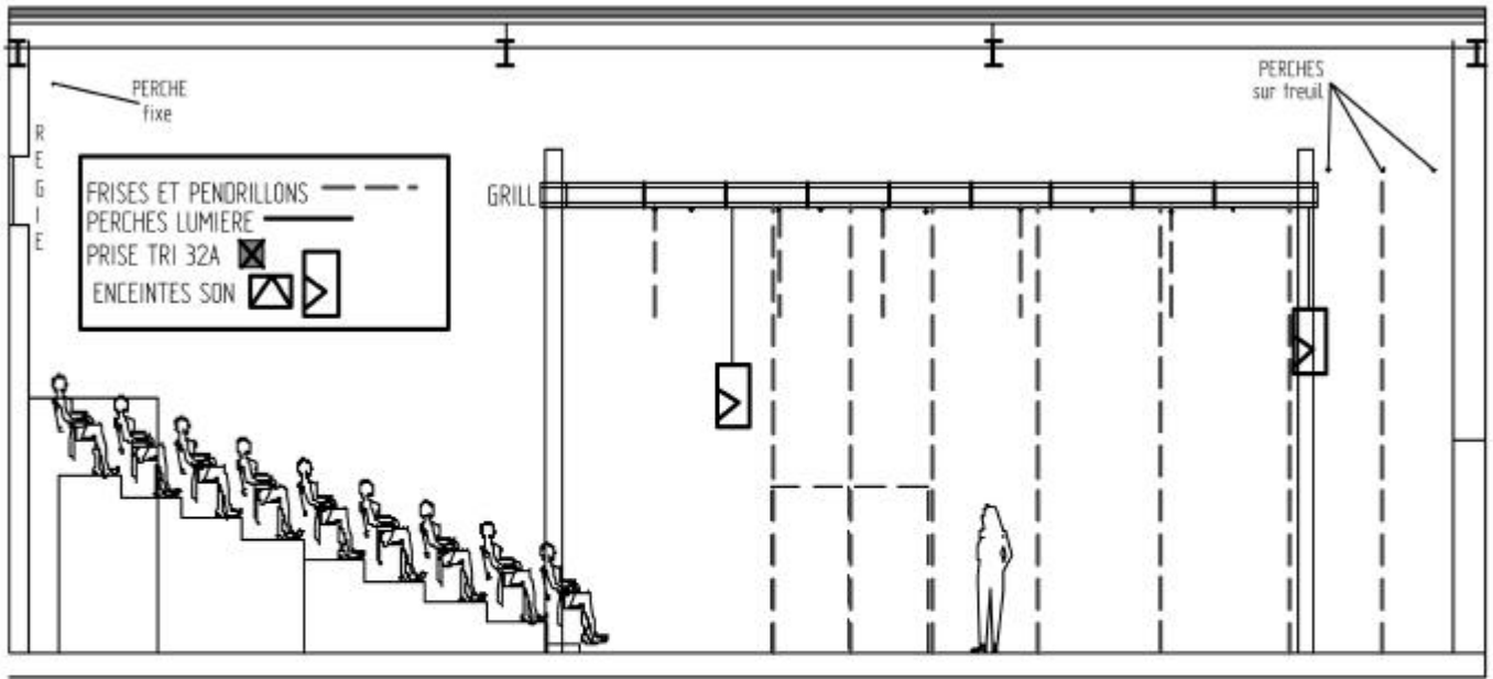
COUPE ET PLAN DE L'ACTEE THEATRE Ech. 100ème
