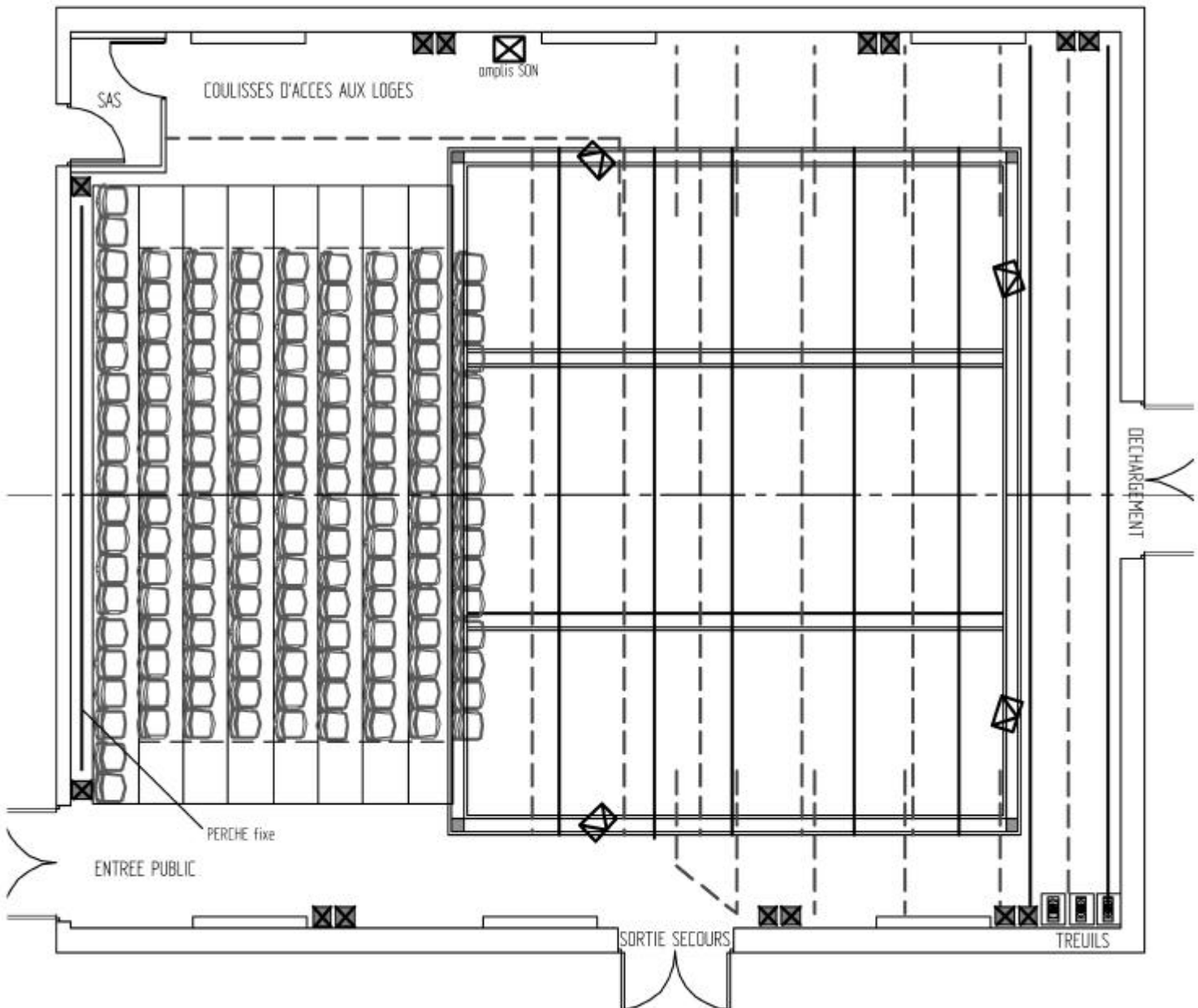
COUPE ET PLAN DE L'ACTEE THEATRE Ech. 100ème
